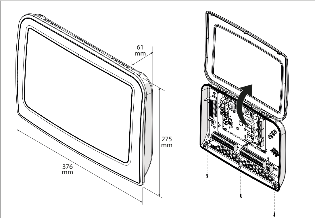
Cotes d'encombrement et dimensions unité intérieure
