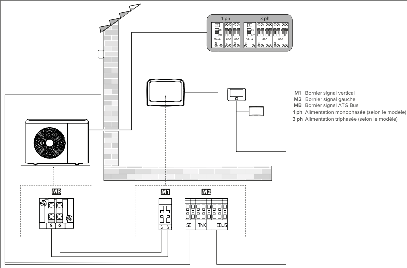
Schéma des raccordements électriques
