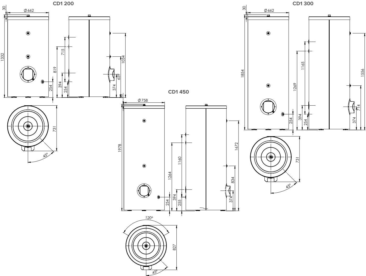
Cotes d'encombrement et dimensions unité intérieure
