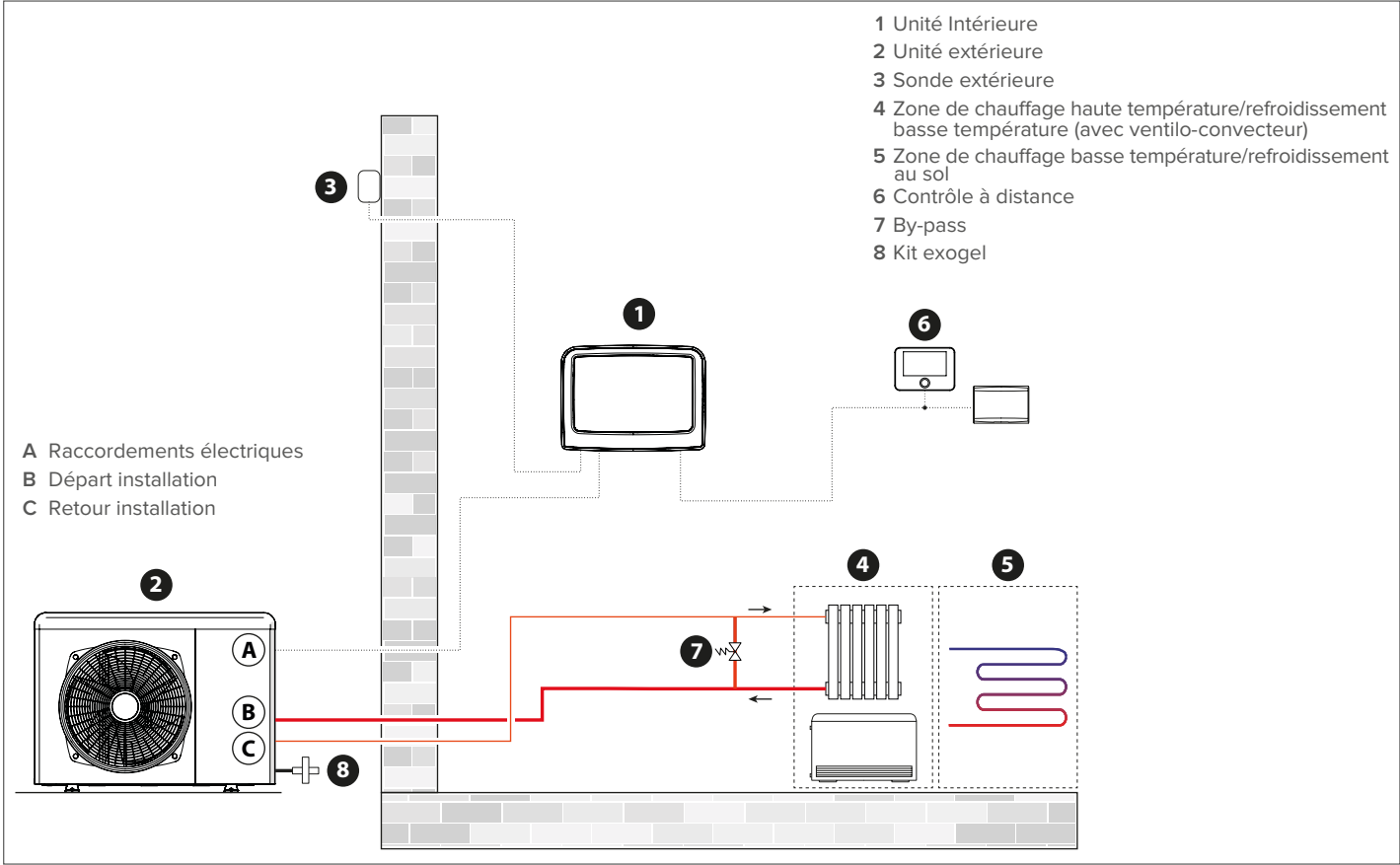
Schéma des raccordements électriques
