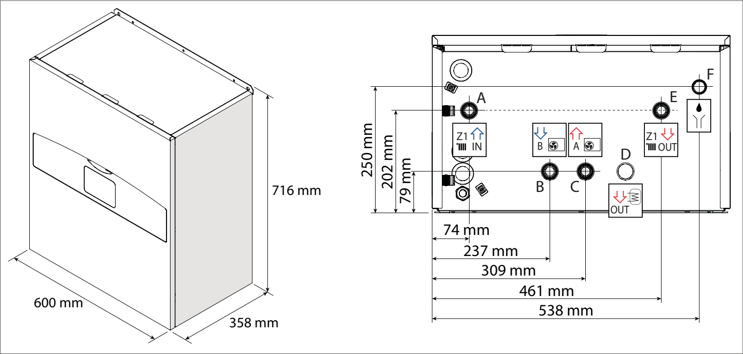
Cotes d'encombrement et dimensions unité intérieure
