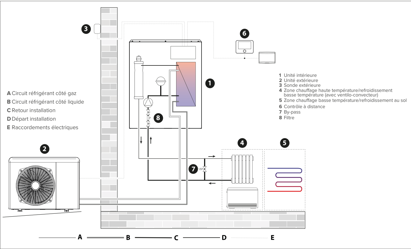
Schéma hydraulique de principe (production ECS par ballon déporté CD1 non représenté)
