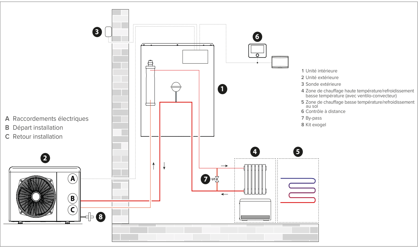
Schéma hydraulique de principe (production ECS par ballon déporté CD1 non représenté)
