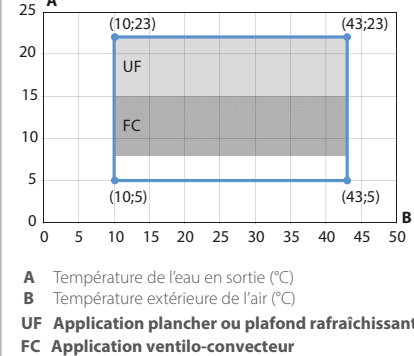
Limites de fonctionnement en refroidissement
