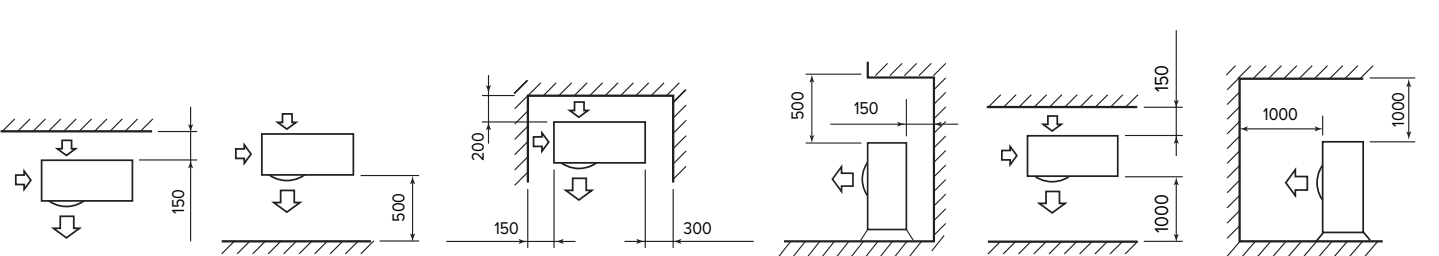
Distances minimales d'installation
