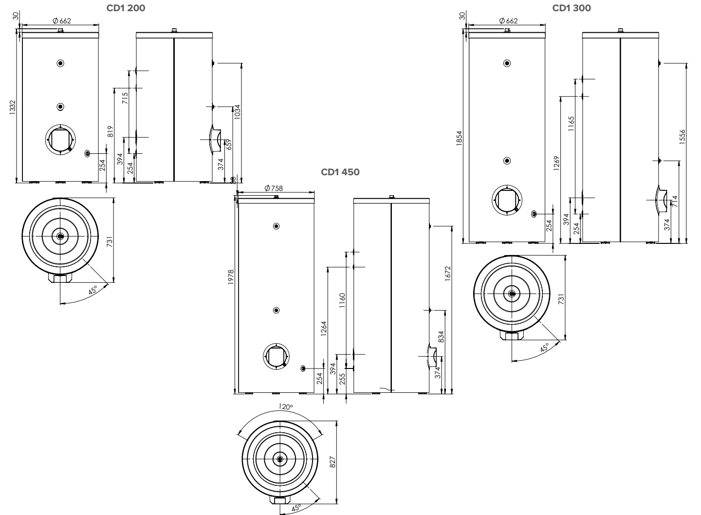
Cotes d'encombrement et dimensions unité intérieure
