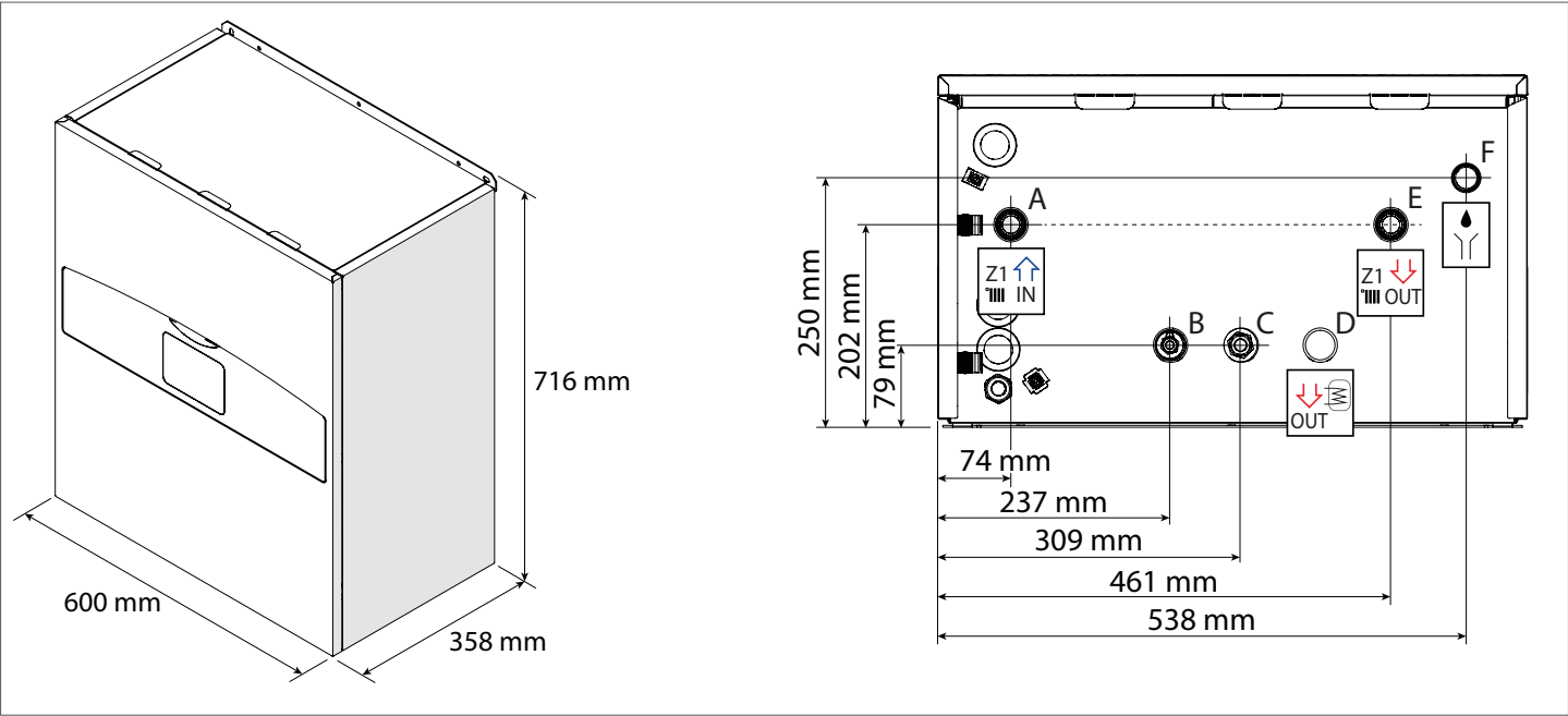
Cotes d'encombrement et dimensions unité intérieure
