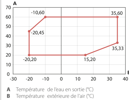
Limites de fonctionnement en chauffage (PAC seule)
