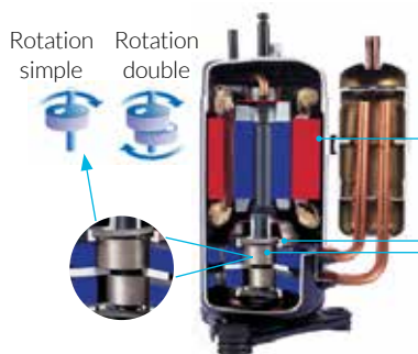
Compresseur rotatif double
